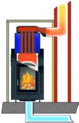
Fonctionnement chaudière avec connection directe
