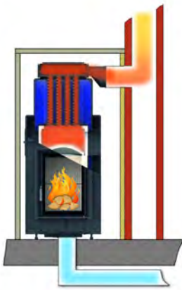
Fonctionnement chaudière avec connection directe
